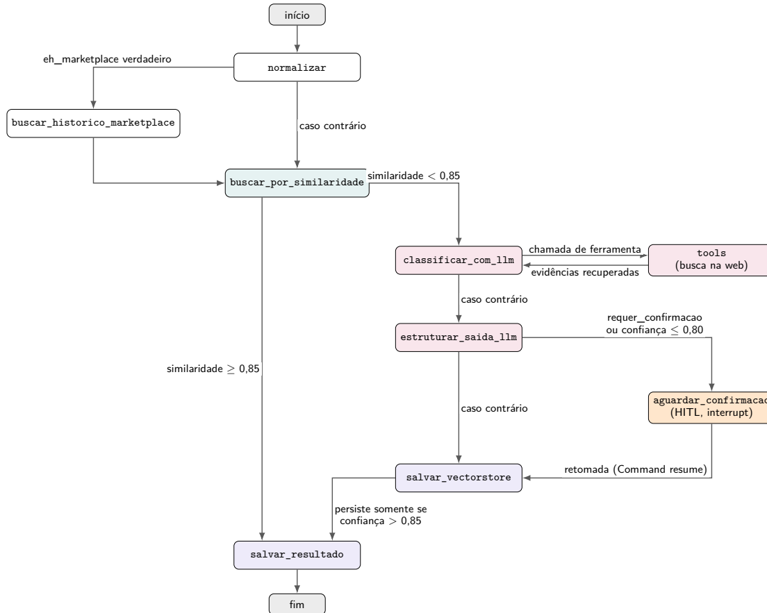
Figura 2 – Grafo de estados do agente de classificação (StateGraph no LangGraph), com a condição de roteamento de cada aresta, conforme codificado na função build_graph .
